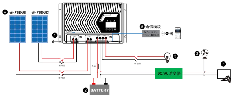
图2-4接线示意图
