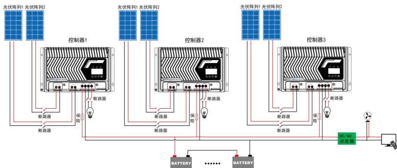
图2-5多机并联接线示意图
