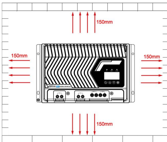
图2-2安装示意图 (IP32)
