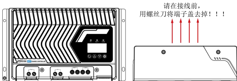
图 2-3 打开端子盖（IP43）
